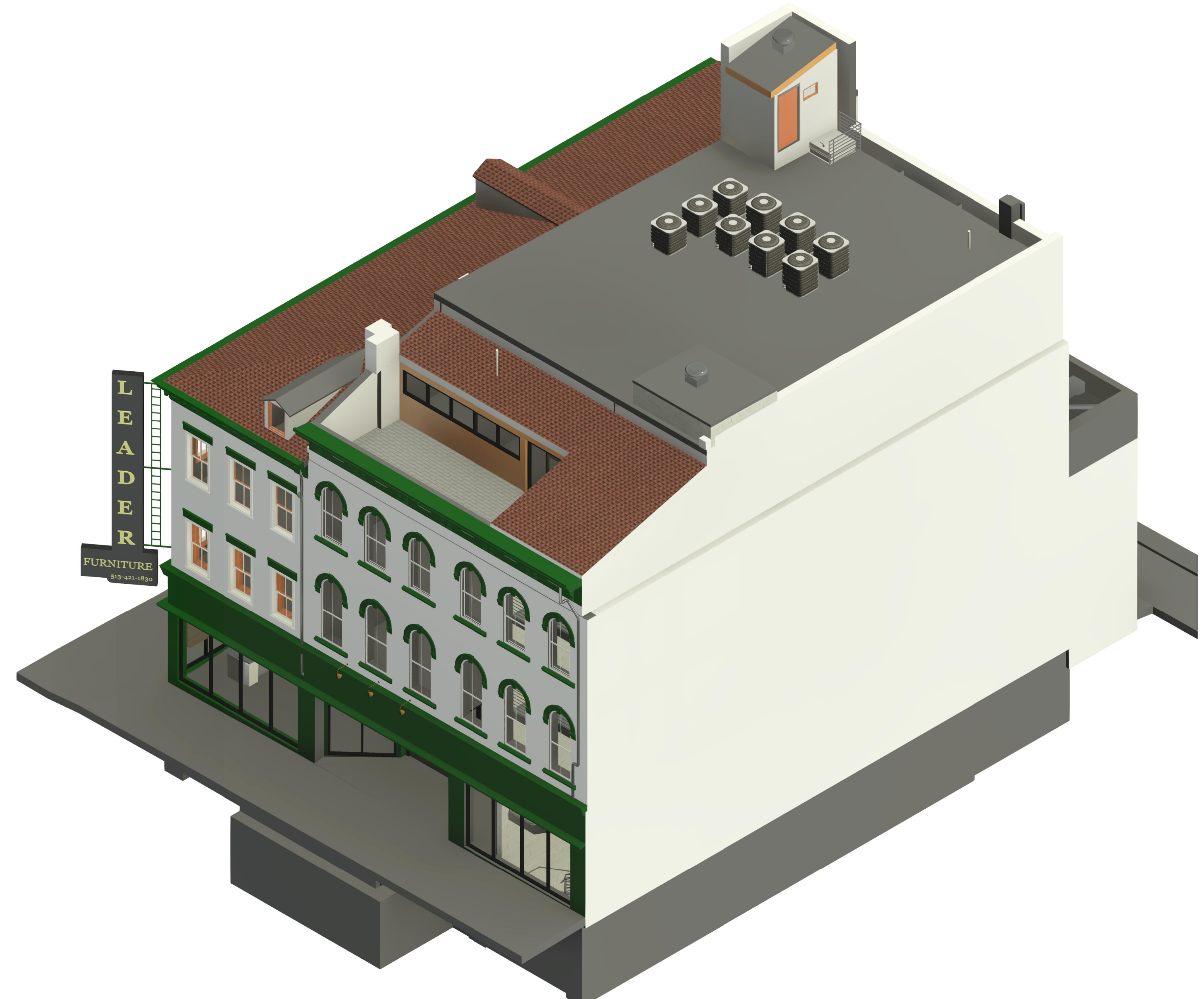
1 3D View SE AXO A2.01
